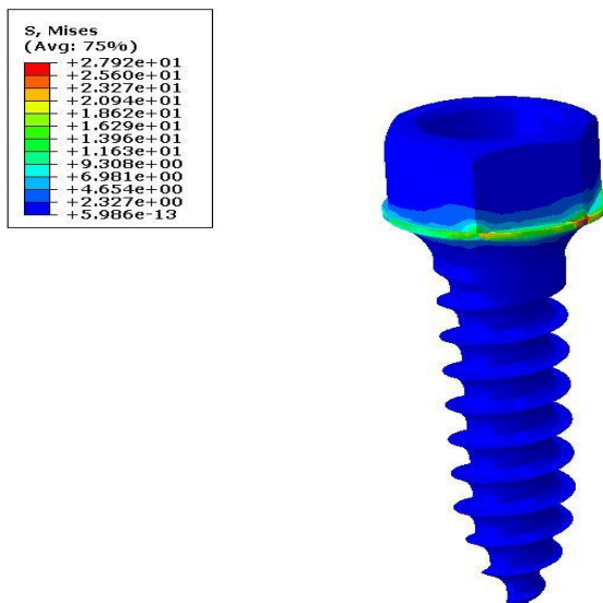
Fig. 3: (d) MiniImplant
